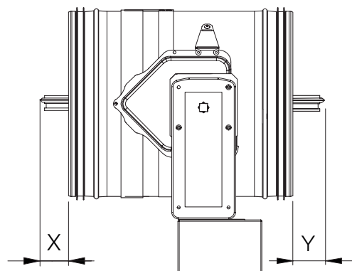
Gehäusetypp für Ex-Elektrischen Federrücklaufmotor und Installationsrahmen
