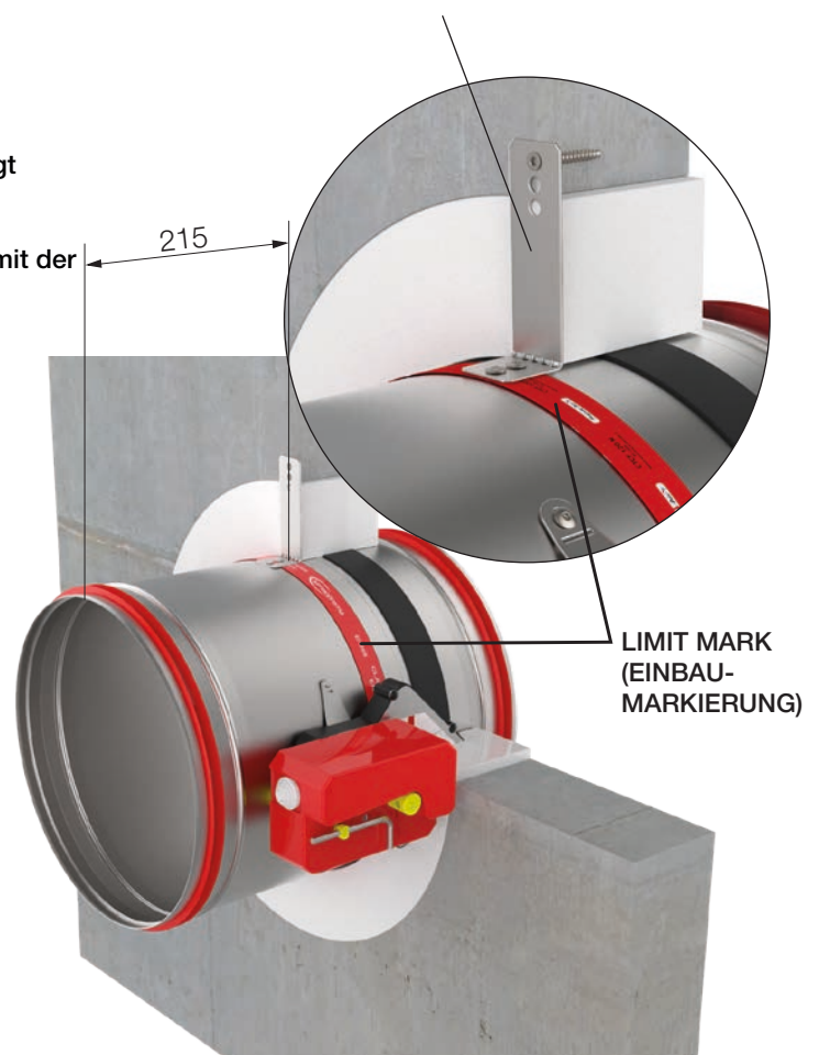
MONTAGEHILFE MIT BEFESTIGUNGSWINKEL
